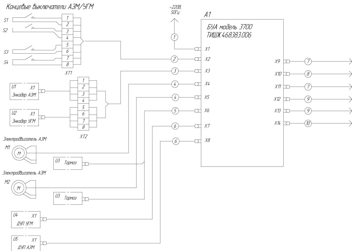
Рисунок 8 - Схема соединений БУА
