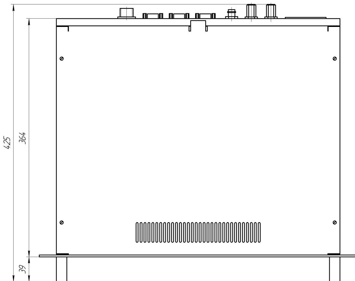
Рисунок 3 - БУА, передняя панель, вид сверху. Габаритные и установочные размеры.
