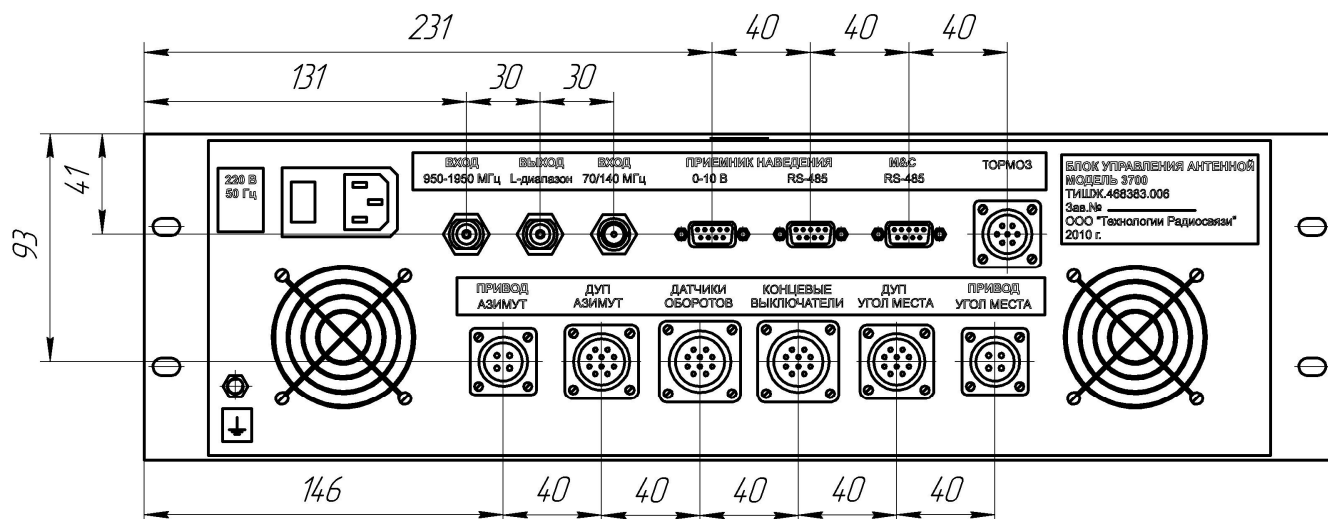
Рисунок 4 - БУА, задняя панель. Габаритные и установочные размеры
